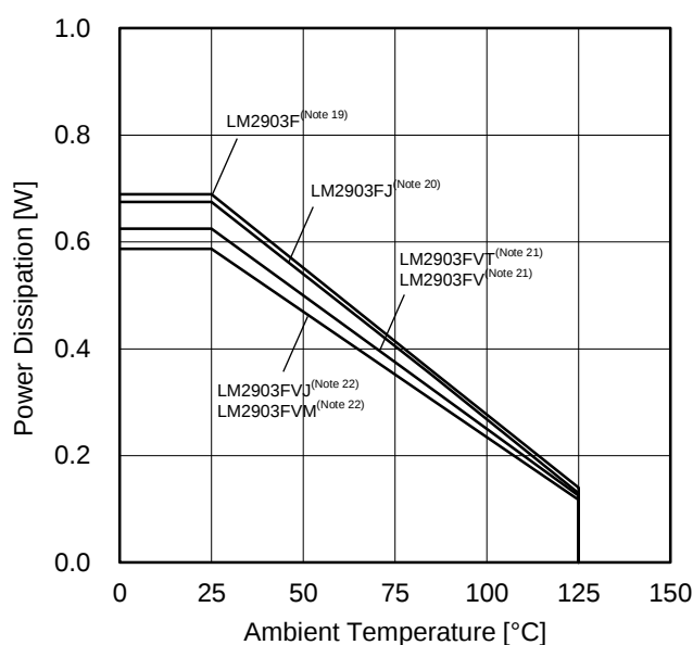
(d) LM2903xxx
